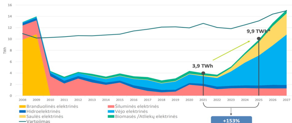
Рис. 4. Динамика производства электроэнергии в Литве в период с 2008 по 2027 год с разбивкой по источникам генерации
