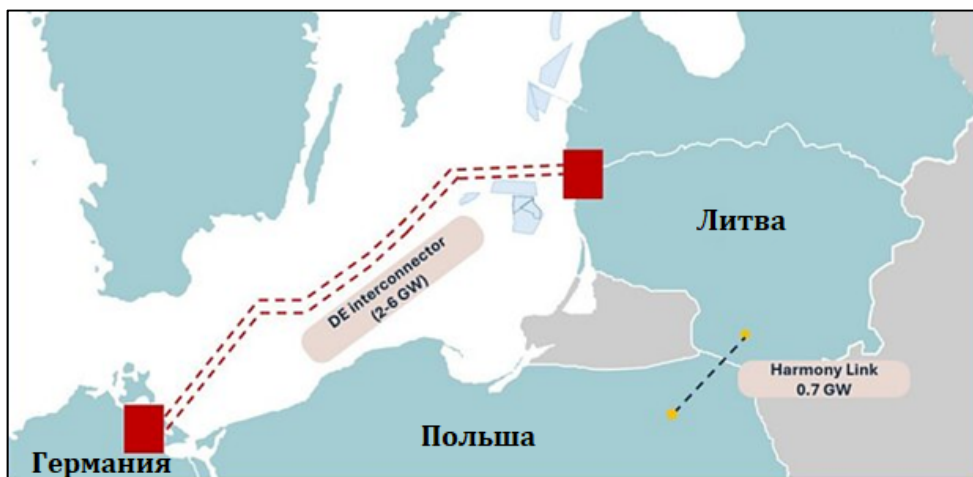
Рис. 2. Схема проекта по прокладке электрического кабеля из Литвы в Германию
